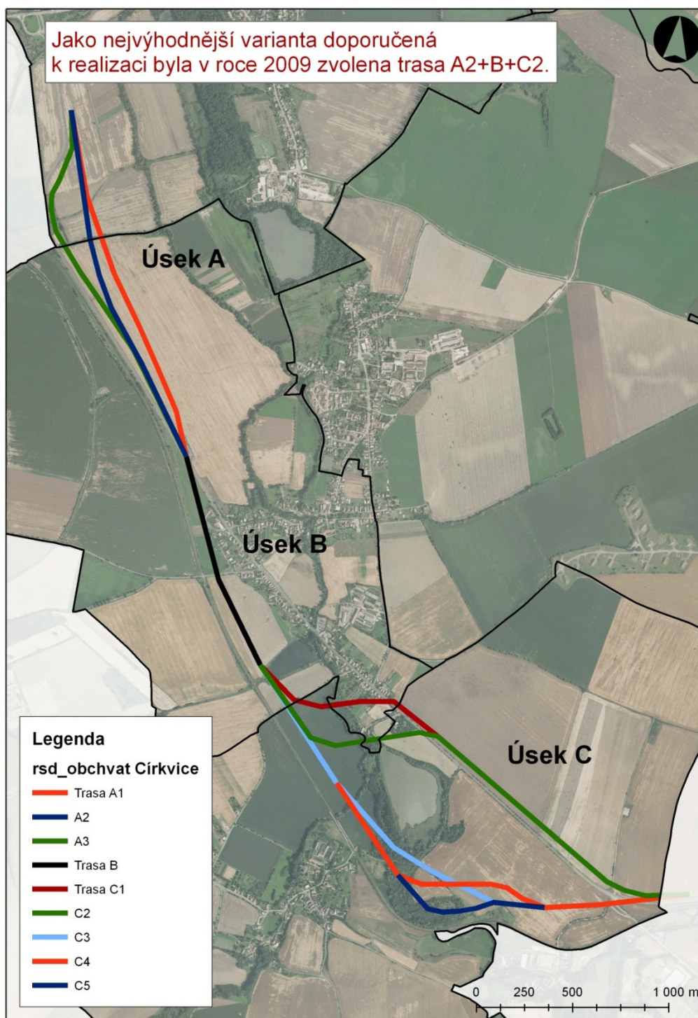
Obr. 3 Variantní řešení obchvatu obce Církvice, zdroj ŘSD ČR, 2009
